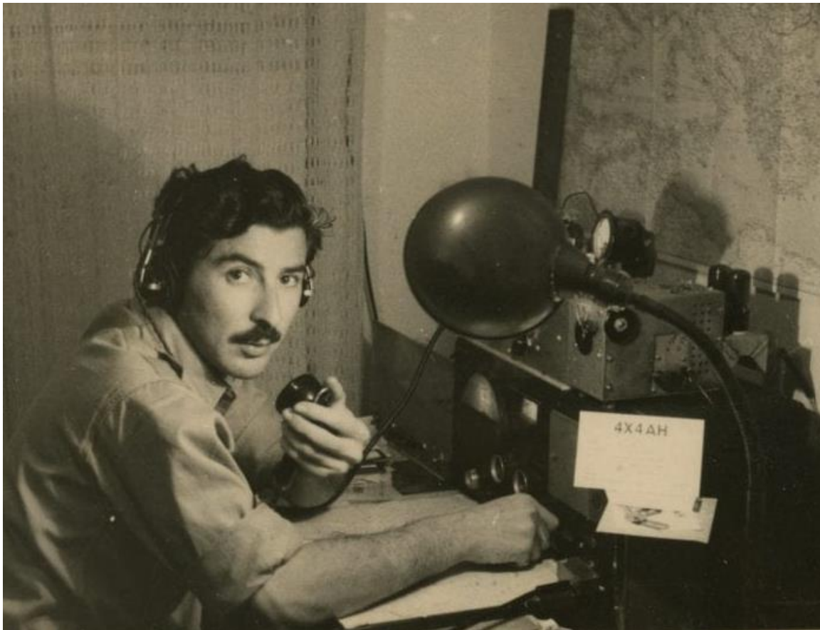
יענקלה יצחק ז"ל, 4X1AH, בתחנת החובבים בביתו בתל אביב, עם מקלט 'הליקרפטר' דגם S.40, ומשדר חובבים מבניה עצמית על בסיס Command Set באדיבות העמותה להנצחת מורשת לוחמי חירות ישראל (לח"י)
