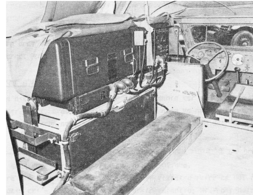
מק-708 בזחל"ם עם קפ-618 ואג-618
