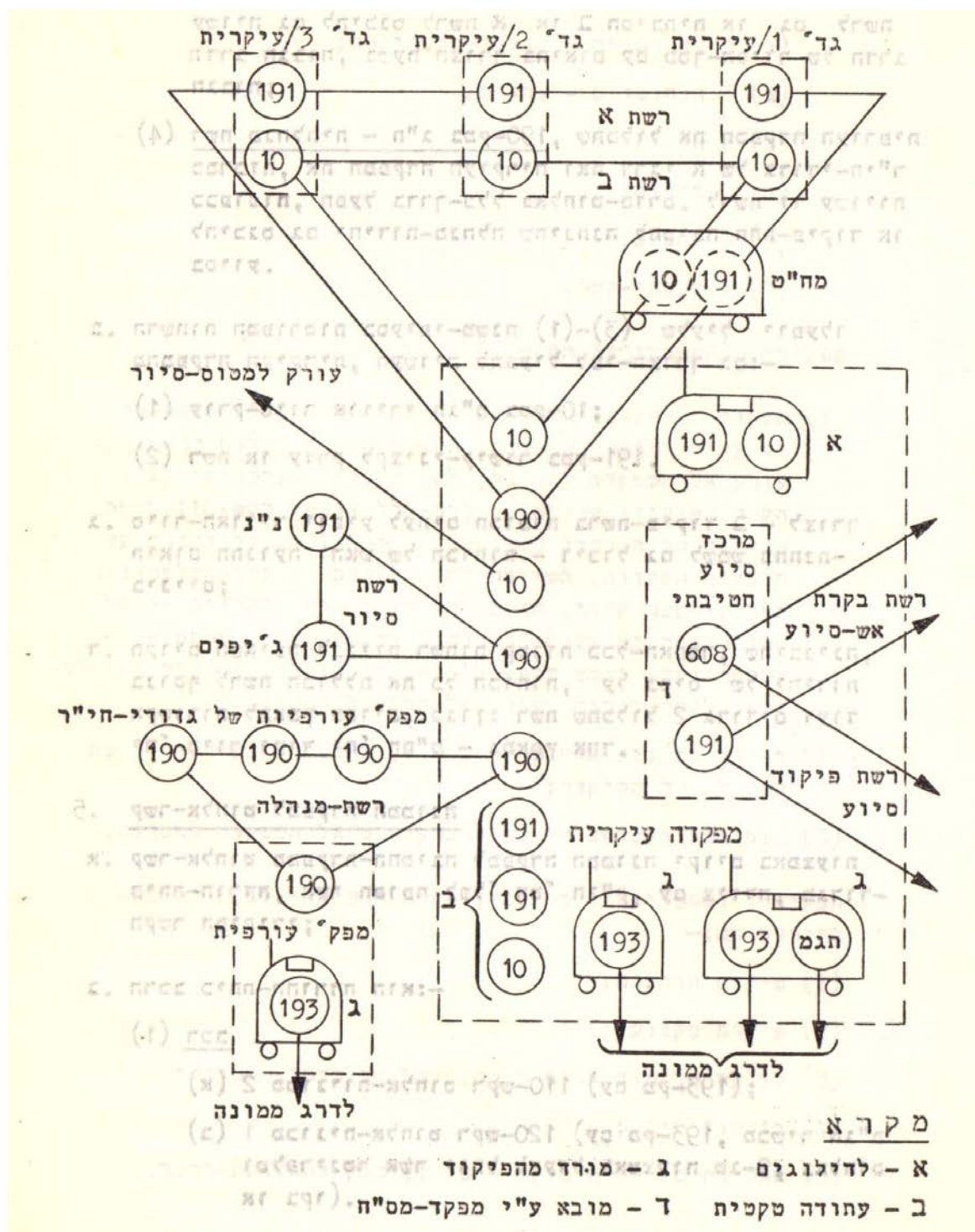
מרשם קשר רדיו חטיבת חי"ר, מוסבת למק-10
