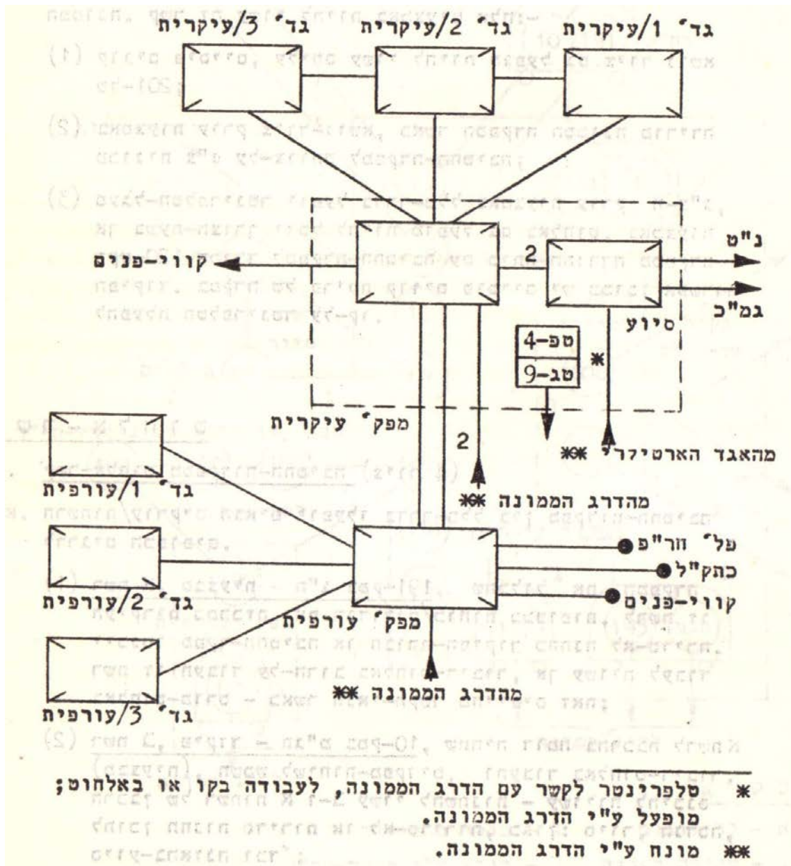
מרשם קשר קווי – חטיבת חי"ר
