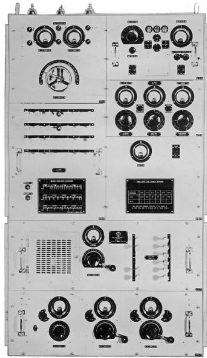
Wireless Set No. 5 בשימוש חיל הקשר הבריטי משנת 1934. משדר בהספק 2,000 ואט, לתחום התדרים 3 עד 30 מה"ץ הדגם שהופעל בארץ שידר בהספק של 500 ואט
