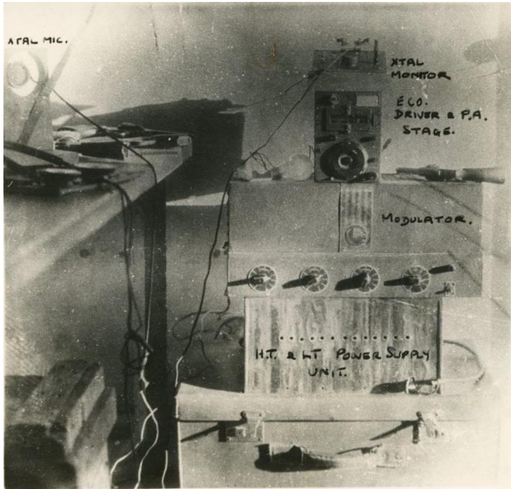
משדר של הלח"י שנתפס בידי הבריטים בפברואר 1946 צילום בריטי. באדיבות העמותה להנצחת מורשת לוחמי חירות ישראל (לח"י)
