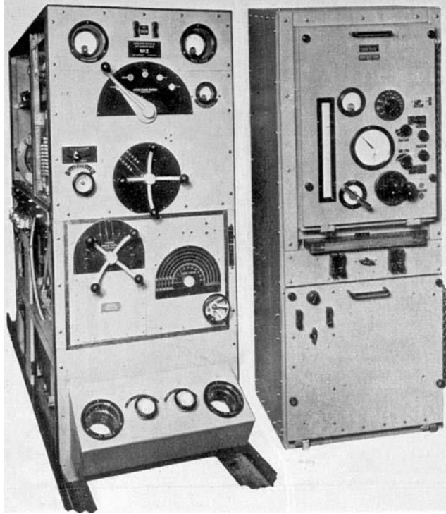
Wireless Set No. 16 בשימוש חיל הקשר הבריטי משנת 1940. משדר בהספק 1,500 ואט בתחום התדרים 0.86 עד 7.6 מה"ץ
