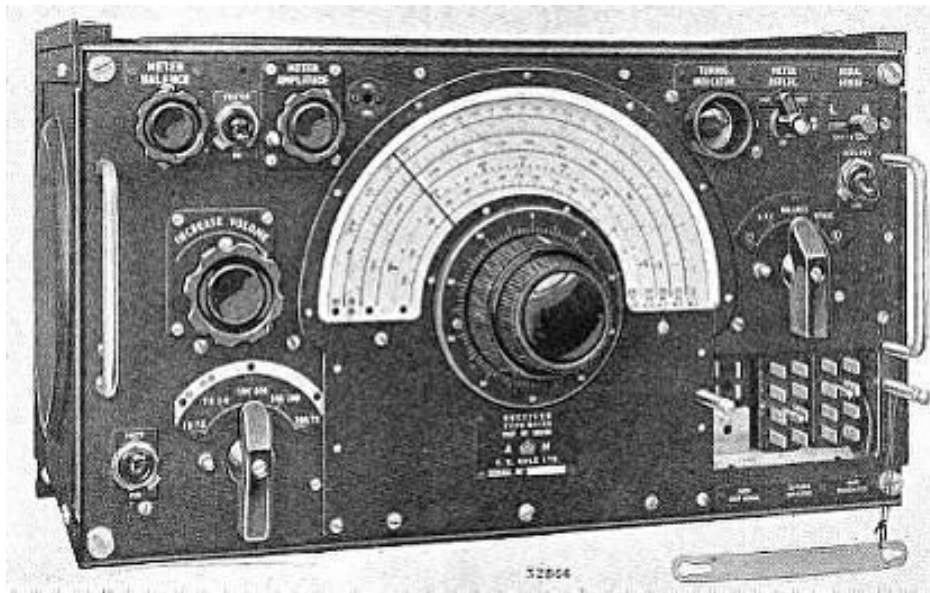
מקלט ת"ג תקני בריטי R.1155, עם מגלה כיוון (DF) מקור: Air Publication 2548A
